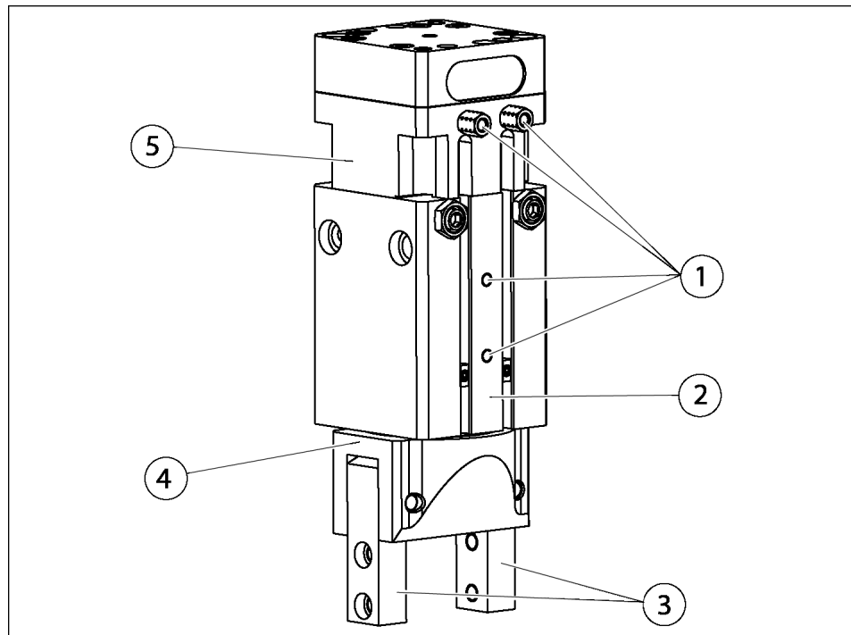
Greif-Schwenk-Modul mit Radialgreifer
