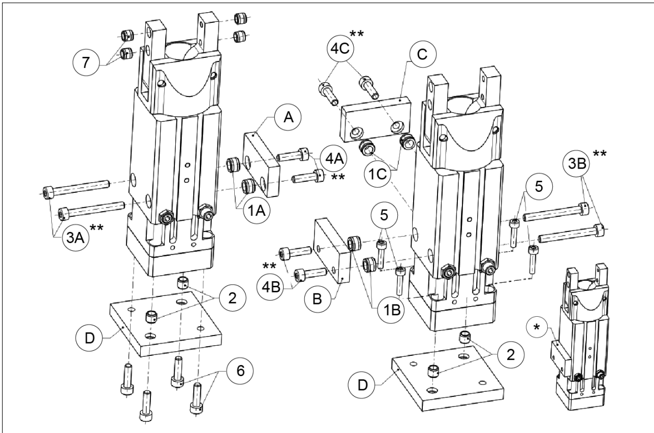
Seitliche und bodenseitige Befestigung des GSM
