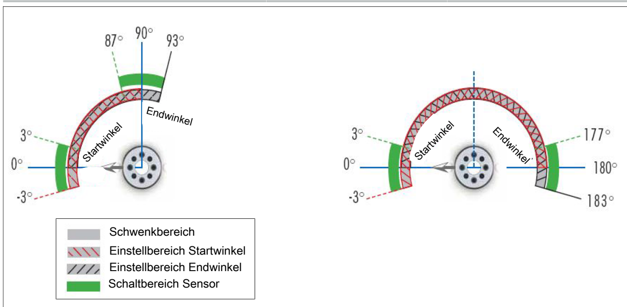
Schwenkwinkeleinstell- und -abfragebereich mit GSM-R
