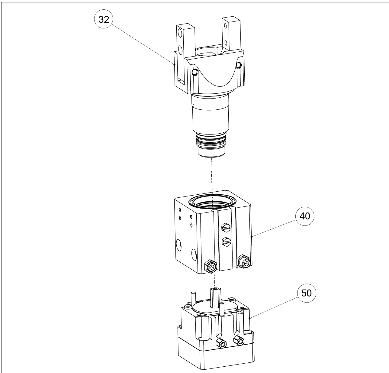
Zusammenbauzeichnung der Grundmodule
