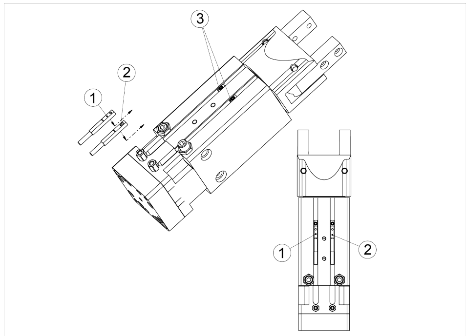
Position und Einbau der Magnetschalter MMS-P
