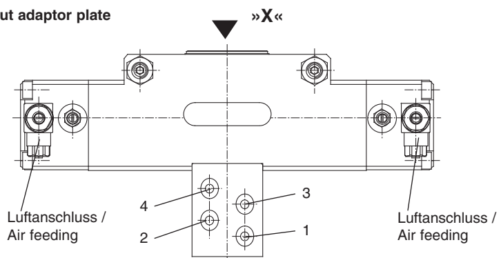
Ansicht »X« / View »X«
