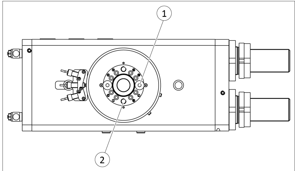
Montageschnittstelle Anbauteil
