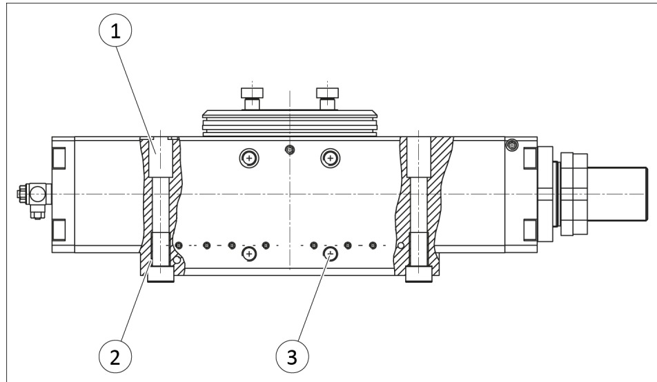
Montageschnittstellen
