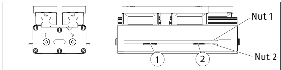
Positionieren der Magnetschalter
