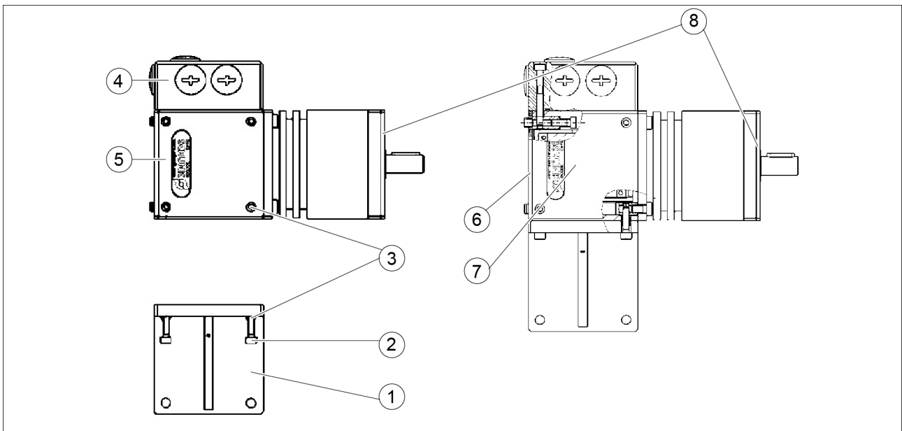
Modul mit Verbindungselement PAM Winkel
