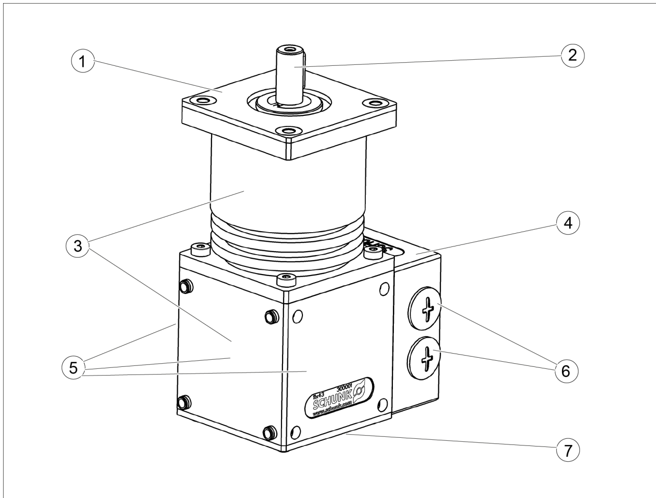
Servoelektrischer Antrieb PDU 2
