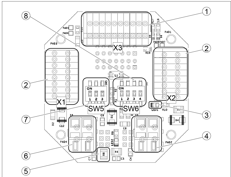
Anschlussplatine
