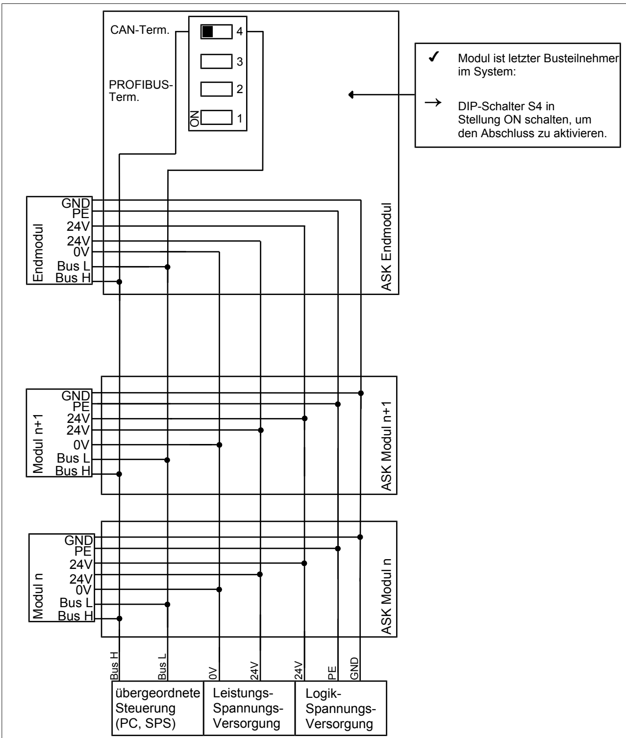
Schaltplan CAN
