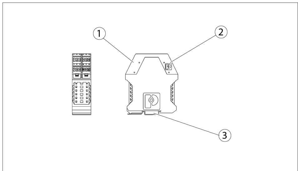
Befestigung MEG C 40
