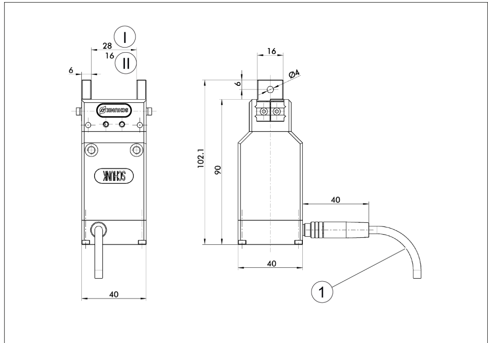
Abmessungen MEG 40 EC (Biegeradius 5xD gilt bei SCHUNK-Anschlusskabel)
