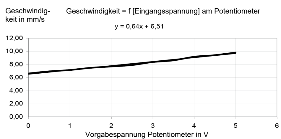
Geschwindigkeit in Abhängigkeit von Eingangsspannung am Potentiometer „Geschw.“ (Potentiometer P2)
