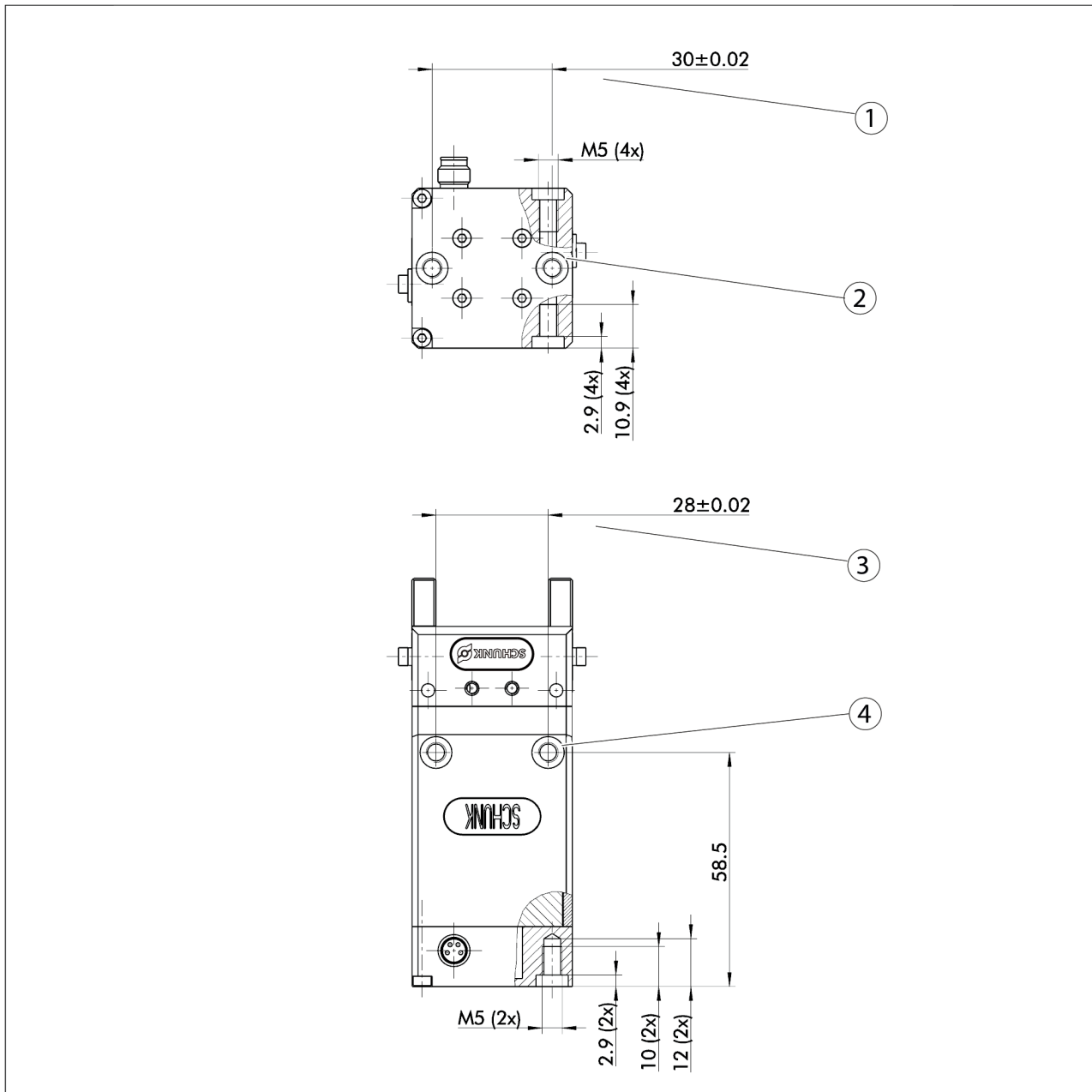
Anschlussmaße MEG 40 EC
