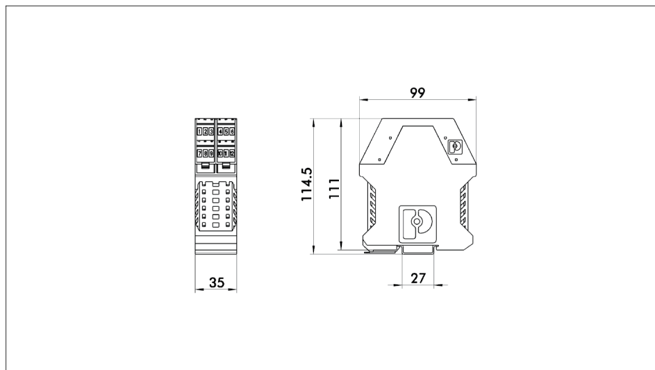
Abmessungen MEG C 40
