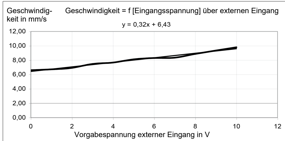
Geschwindigkeit in Abhängigkeit vom externen Analogeingang „Geschwindigkeit“ (Klemme 22)
