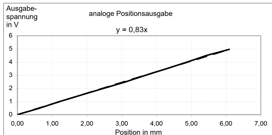
Zusammenhang zwischen analoger Positionsangabe (Klemme 15) und Position des Greifers
