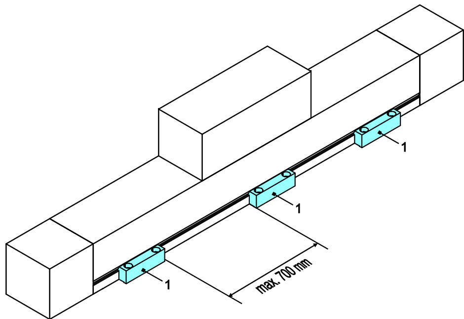
Bild 4: Befestigungsleisten(1)
