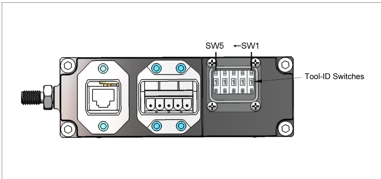
DL5 Tool Module, Tool-ID Switch Settings
