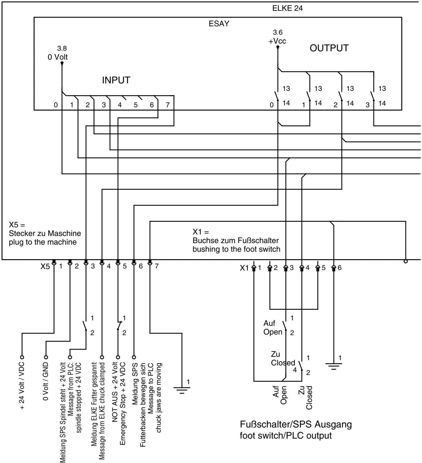
Kunden SPS Anschluss Customer PLC connection
