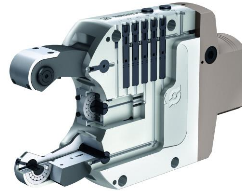
Zentralschmierung
