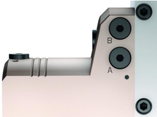
Seitliche Hydraulikanschlüsse
