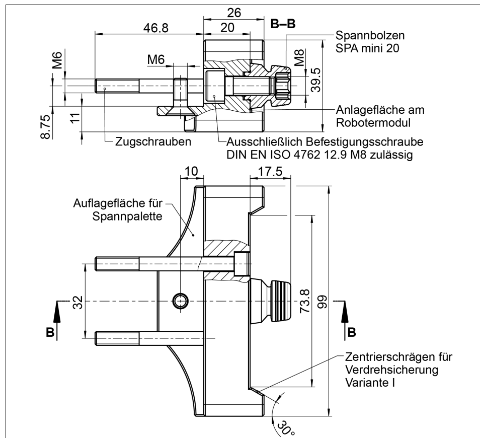
Palettenkupplung PKL mini 100
