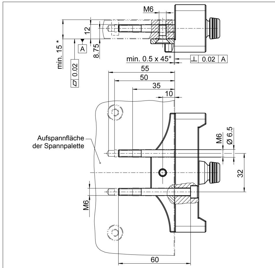
Verbindungsschnittstelle zwischen Spannpalette und Palettenkupplung
