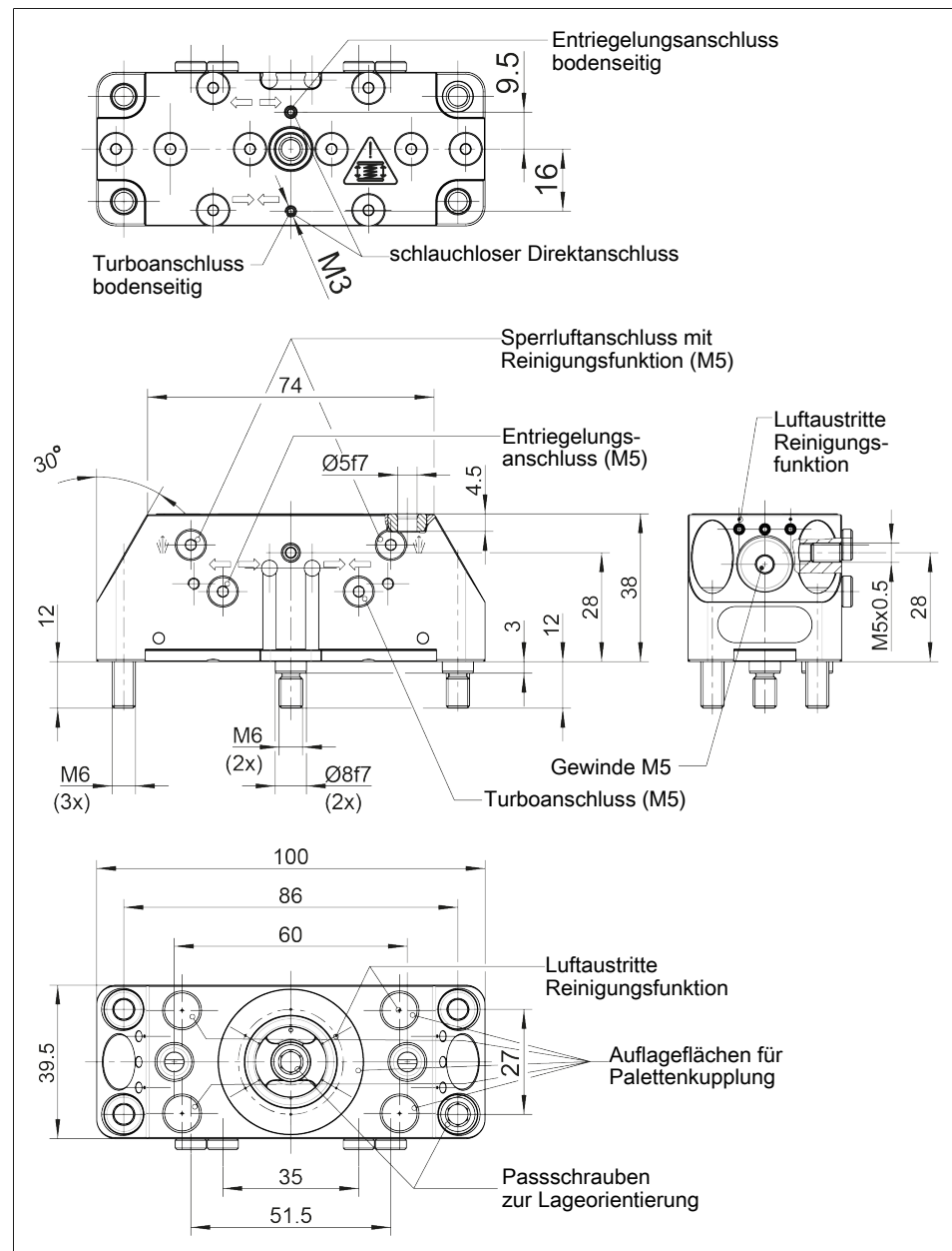
Befestigung und Anschlüsse
