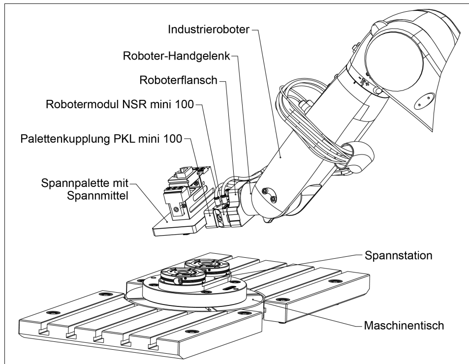
Anwendungsbeispiel für die automatisierte Palettenbeladung
