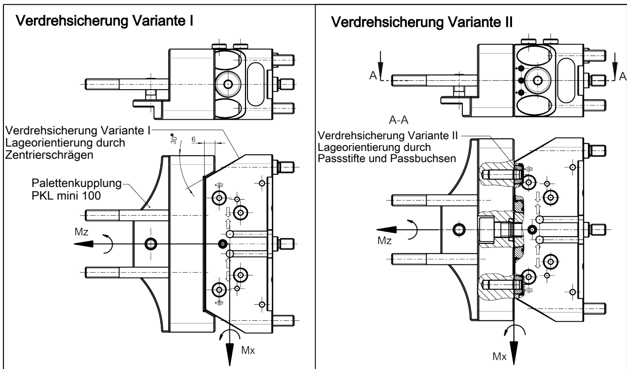
Verdrehsicherung Variante I und Variante II
