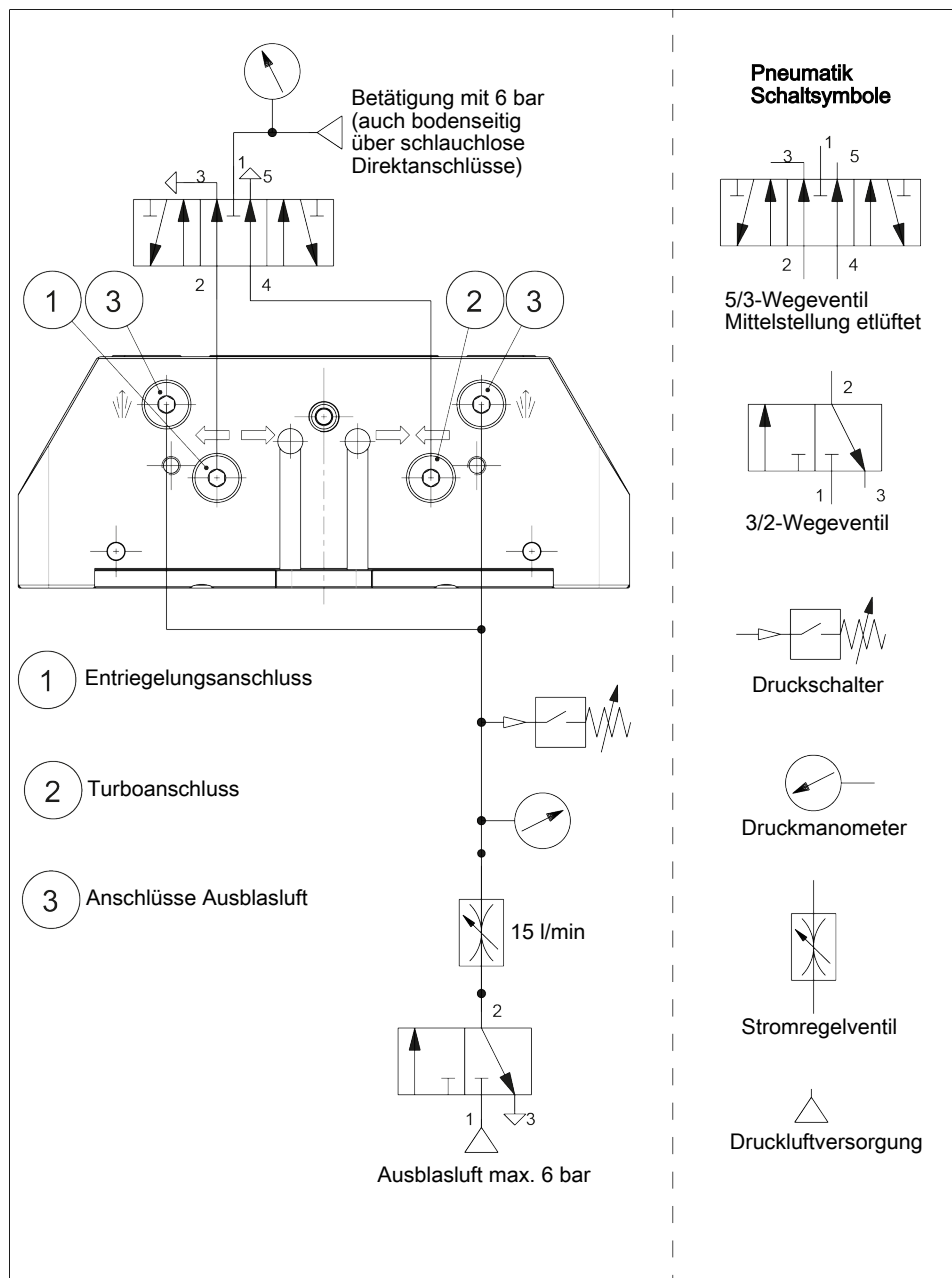
Pneumatik-Schaltplan
