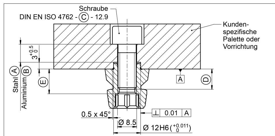
Toleranzen und Einbaubedingungen für Spannbolzen SPA mini 20
