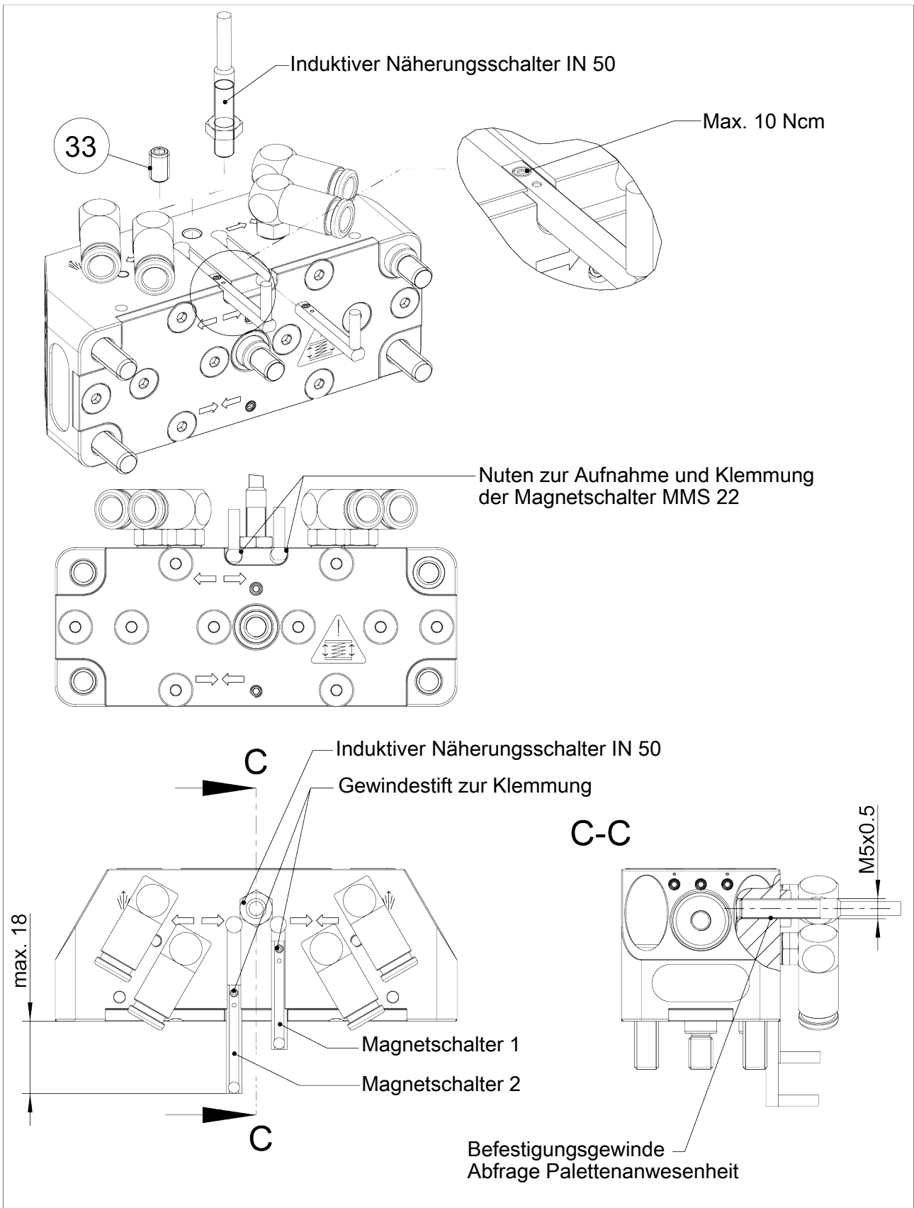
Montage der Näherungsschalter
