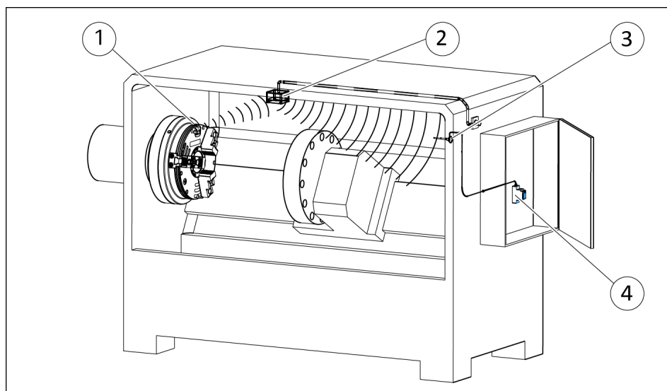
Beispielhafte Anordnung der Antenne und des Repeaters
