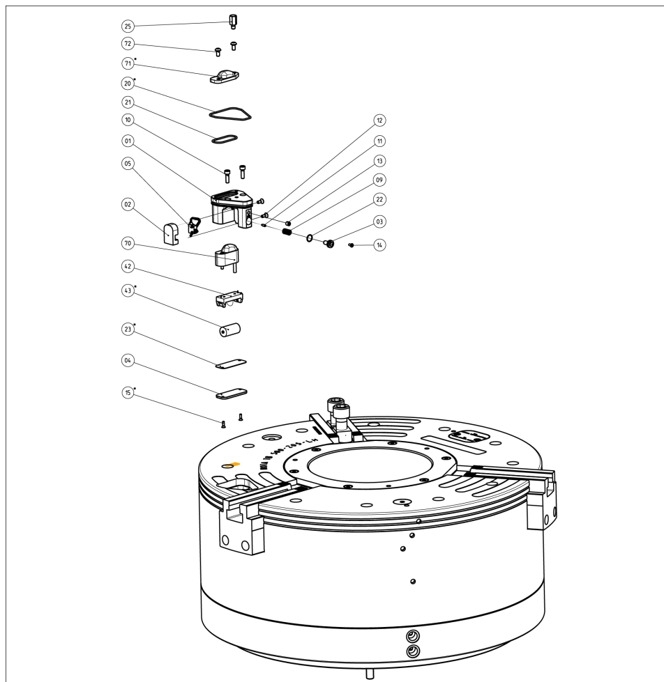
Zusammenbau ROTA TB/EP
