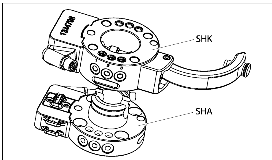
Bohrbild nach DIN ISO 9409-1, Prinzipskizze
