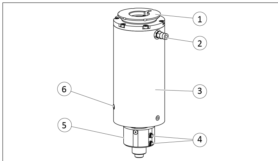
Axial und radial nachgiebiges Entgratwerkzeug mit automatischem Werkzeugwechsel
