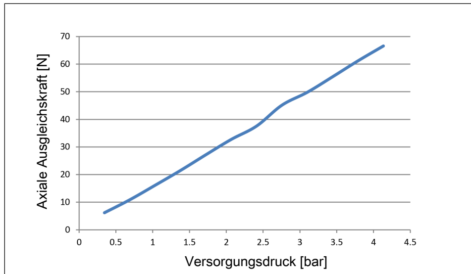
Axiale Ausgleichskraft in Abhängigkeit zum Betriebsdruck
