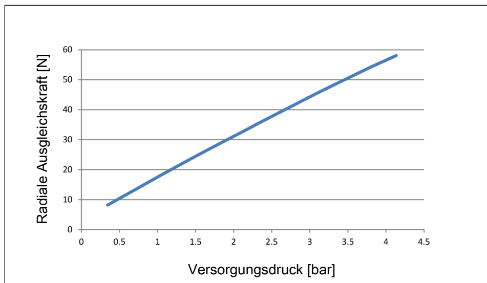
Radiale Ausgleichskraft in Abhängigkeit zum Betriebsdruck
