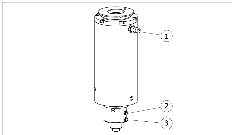
Variante CDB-ATC mit automatischem Werkzeugwechsel
