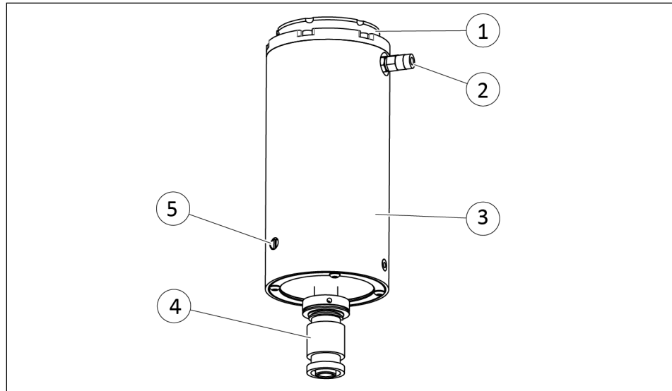
Axial und radial nachgiebiges Entgratwerkzeug mit manuellem Werkzeugwechsel
