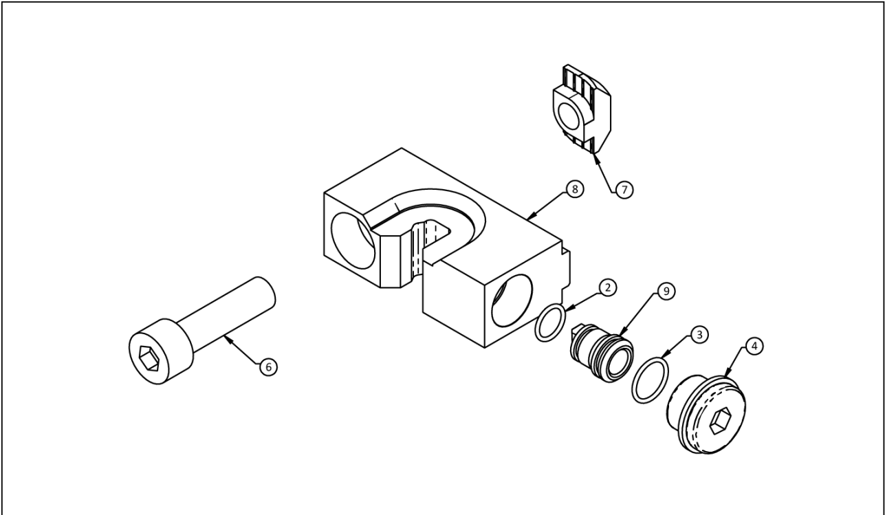
Tool stand module
