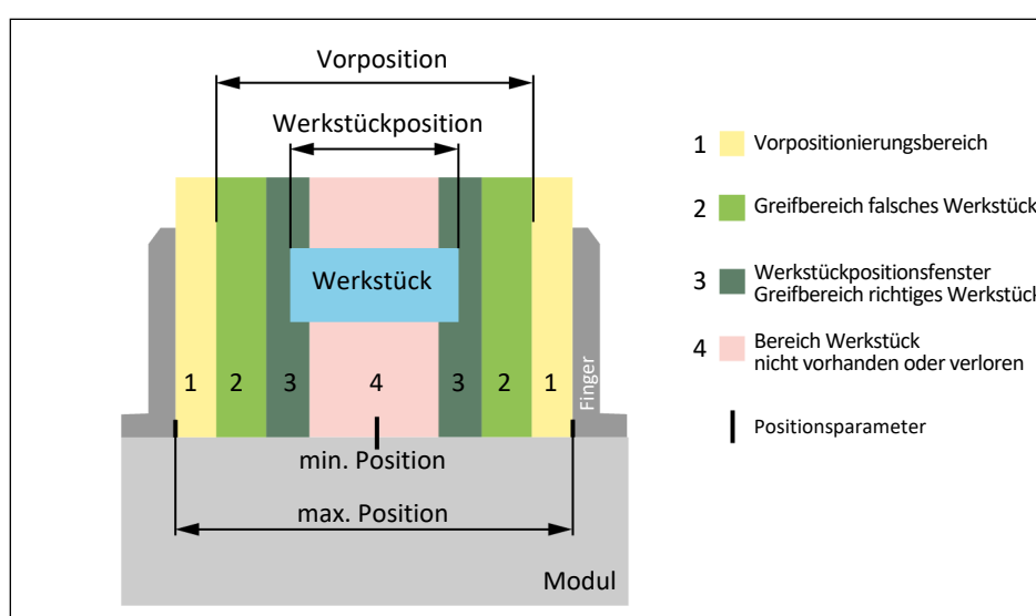
Werkstück greifen an erwarteter Position, Beispiel Außengreifen
