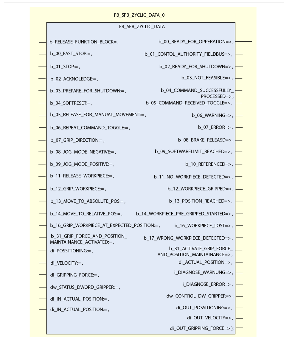
Ein- und Ausgangsdaten für zyklische Kommunikation
