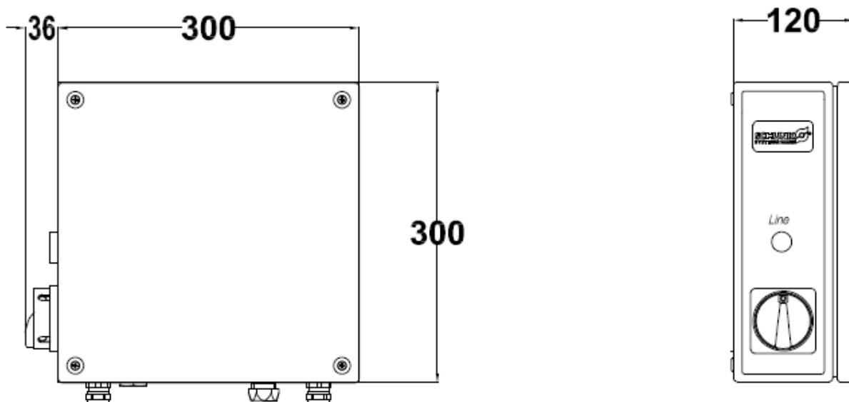
Fig. 5 Ingombri 0420612, 0420606, 0420610, 0420611, 0420604, 0420605, 0420614, 0420608
