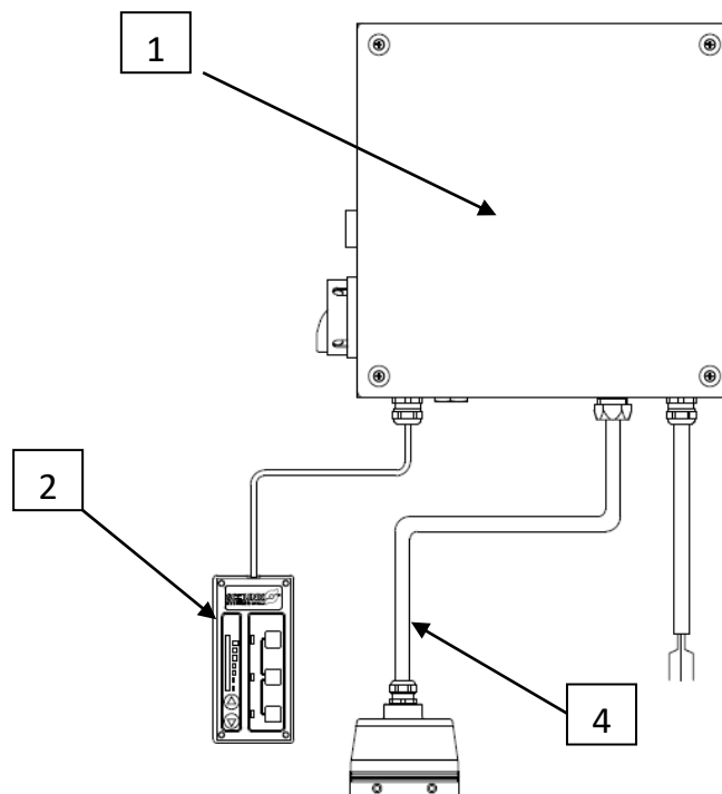
Fig. 1 Versione 0420606, 0420607, 0420612 e 0420613 per piani con connettore circolare
