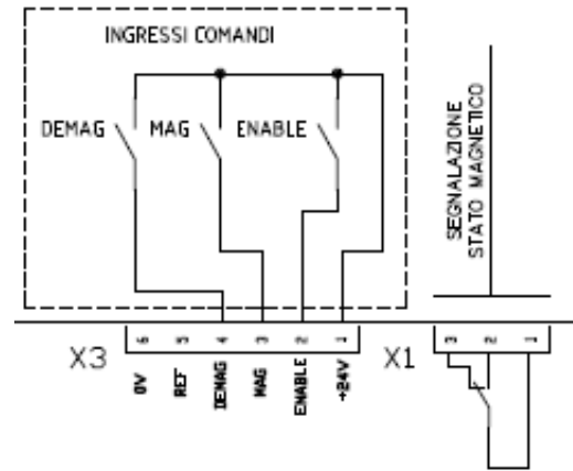
Fig. 12 Connessione raccomandata per le versioni 0420612, 0420606, 0420610, 0420604, 0420612, 0420606
