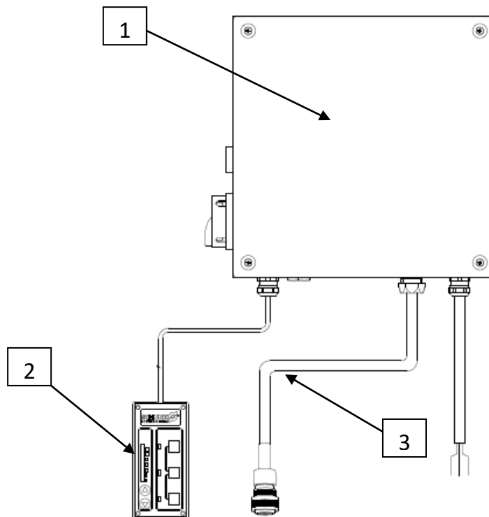
Fig. 1 Versione 0420606, 0420607, 0420612 e 0420613 per piani con connettore circolare
