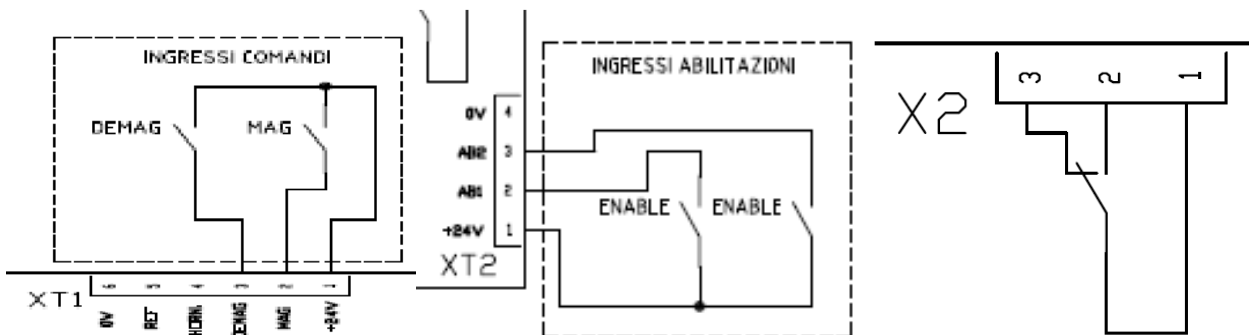
Fig. 13 Connessione raccomandata per le versioni 0420613, 0420607, 0420611, 0420605, 0420615, 0420609
