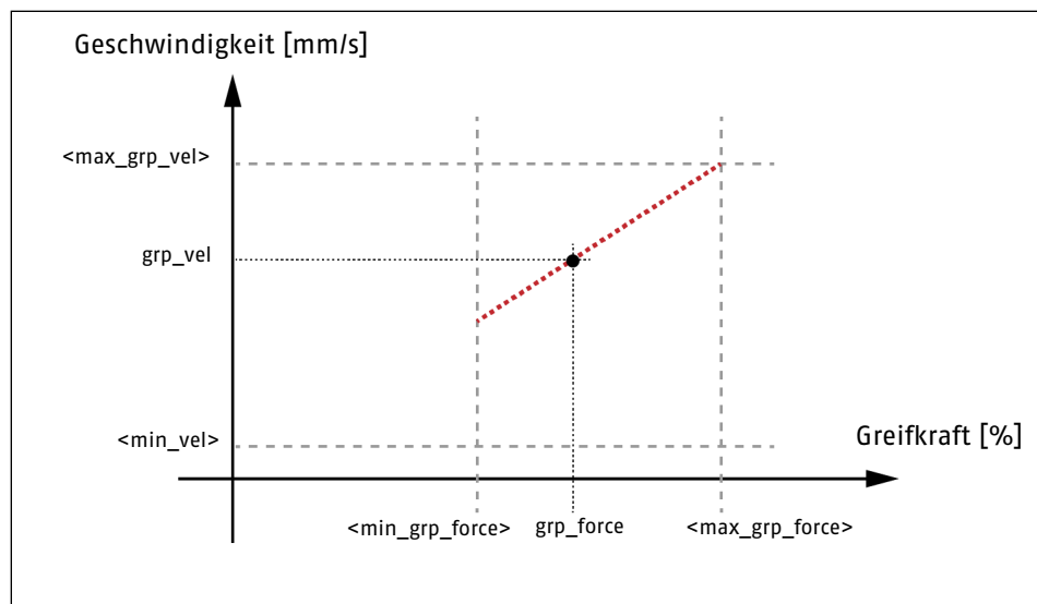
Greifgeschwindigkeit in Abhängigkeit von der Greifkraft
