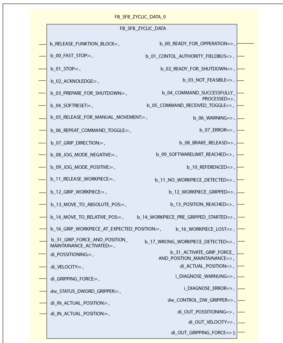
Ein- und Ausgangsdaten für zyklische Kommunikation
