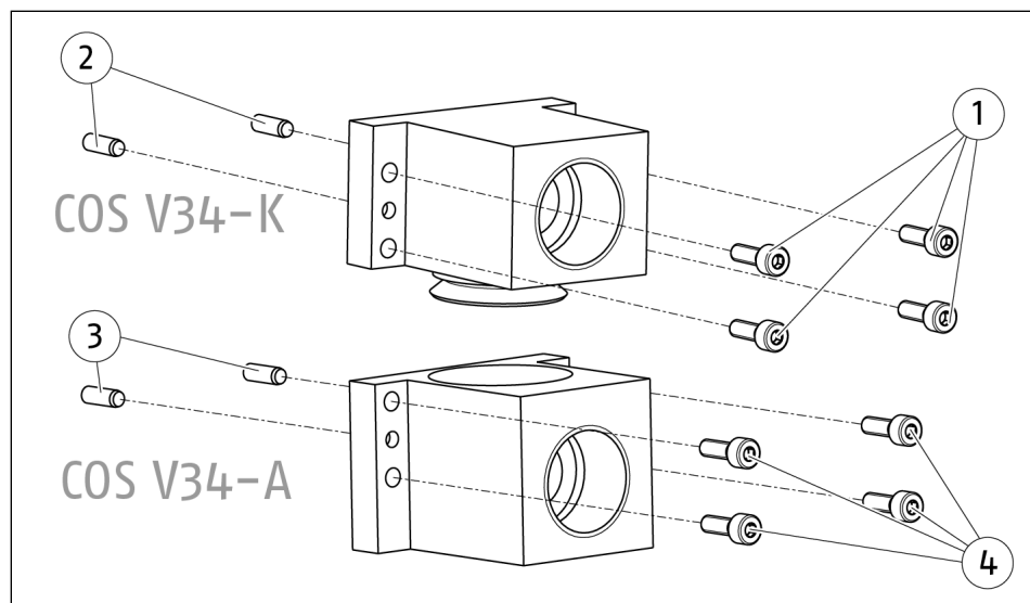
Mounting optional module COS V34
