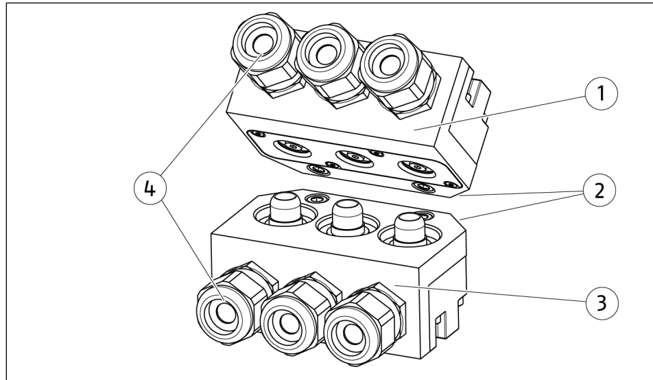
Elektrisches Optionsmodul COS PY 41
