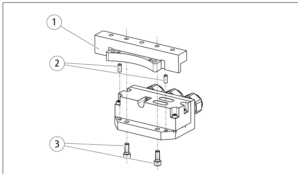
Adapterplatte montieren
