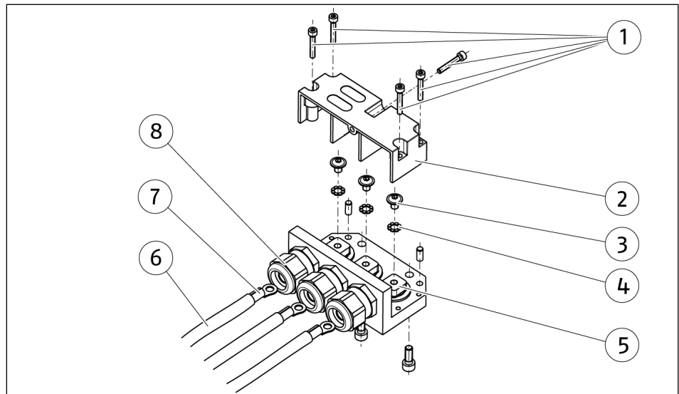
Kabel installieren, dargestellt an COS PY41-K
